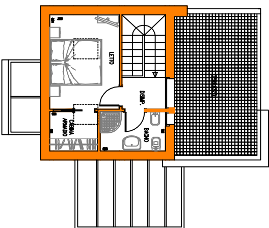
piano secondo
