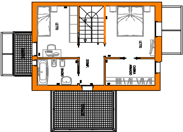
piano primo
